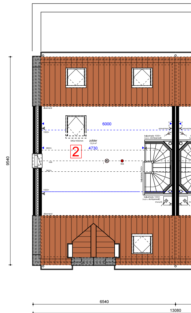
ZOLDER (optie 2)
