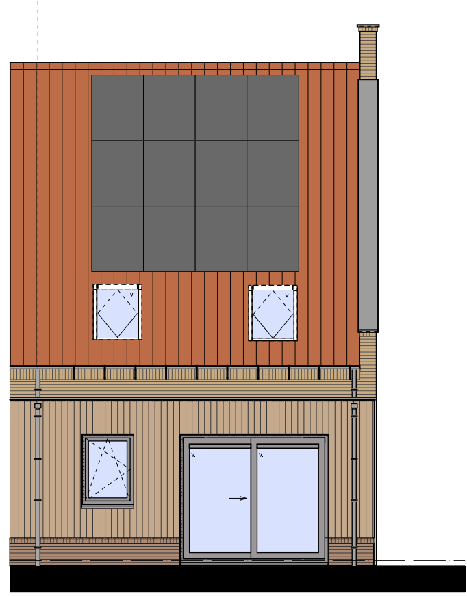
4 ACHTERGEVEL
