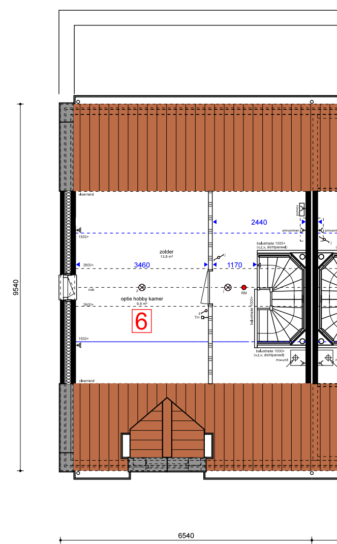
ZOLDER (optie 6)
